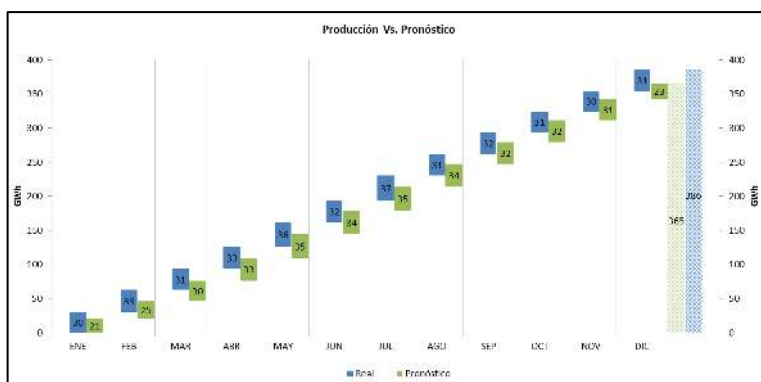
Gráfico 2 Producción mensual acumulada Vs. pronóstico de hidrología media de la central Normandía
