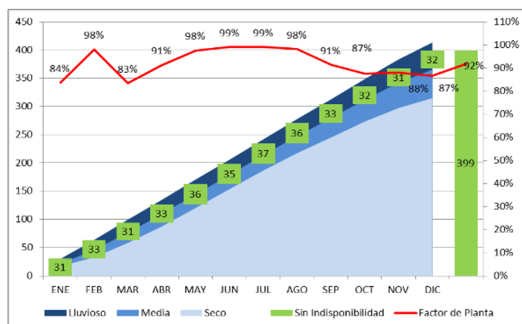
Gráfico 3 Producción mensual acumulada de la central Normand sin indisponibilidades
