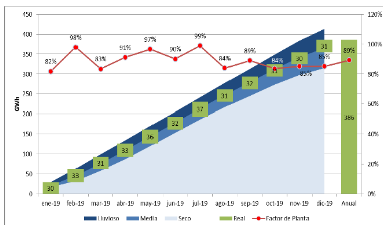
Gráfico 1 Producción mensual acumulada de la central Normandía
